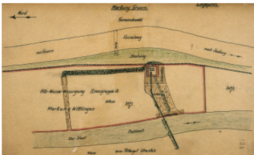
Lageplan der projektierten Quellzuleitung von den Brunnen im Fischbachtal zur geplanten Pumpstation, 1896/1910, aus den Akten zum Ausbau der Albwasserversorgung Ermsgruppe XIII hinsichtlich der Wasserversorgung des Truppenübungsplatzes Münsingen.
