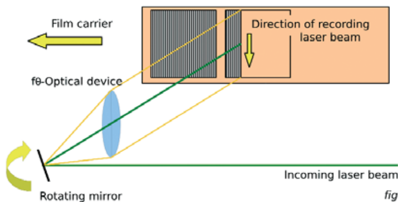
Die Funktionsweise des Laserbelichters.
