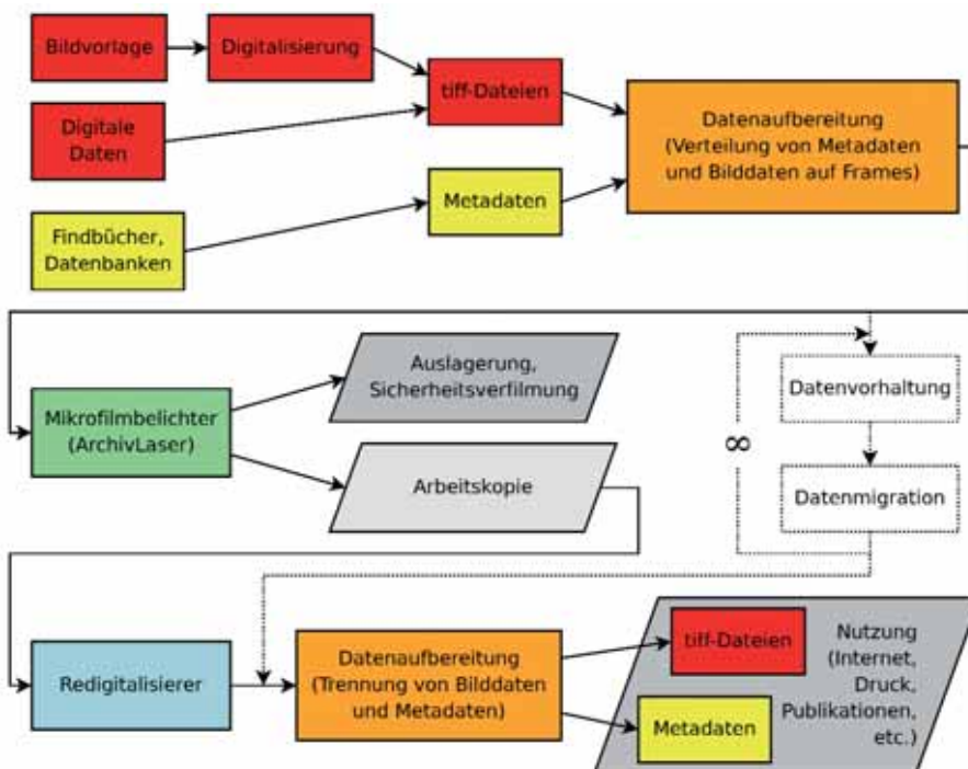
Die schematische Darstellung des ARCHE-Workflows.
