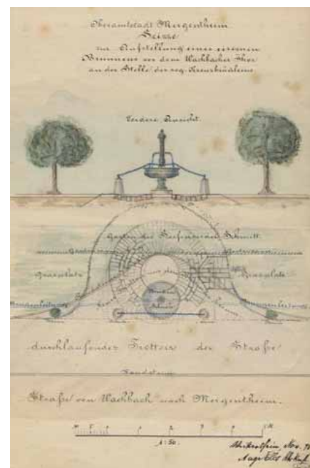
Entwurf eines eisernen Brunnens beim Wachbacher Tor in Bad Mergentheim, kolorierte Zeichnung von 1875. Vorlage: Landesarchiv StAL F 225 II Bü. 27
